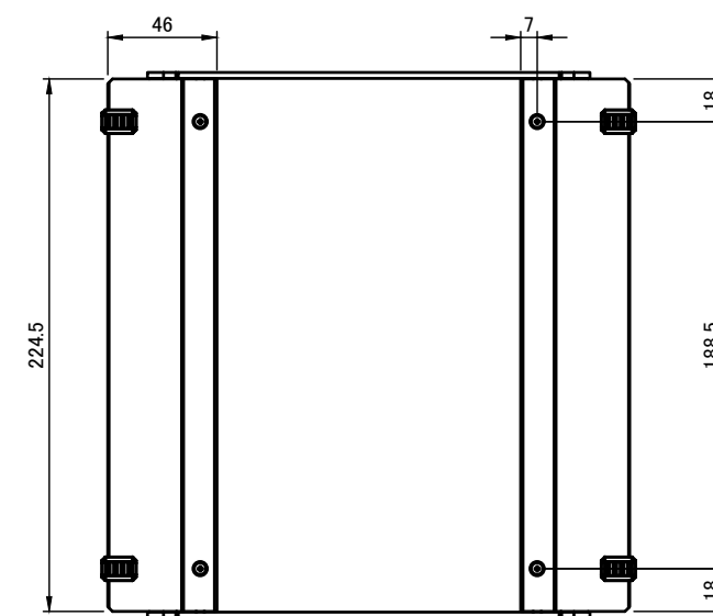
D-D ( 1 : 3.5 )
