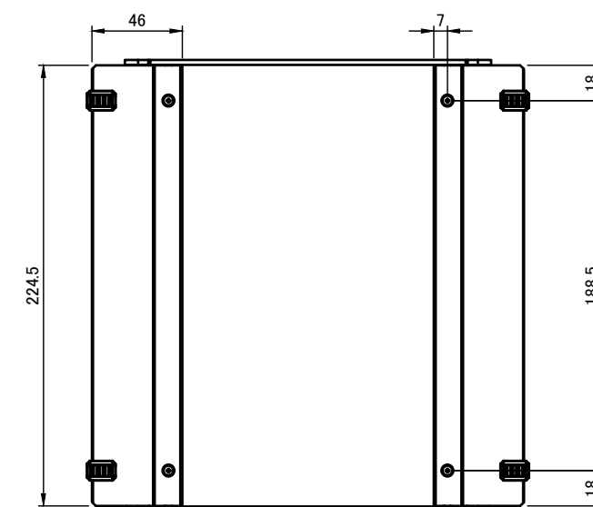
D-D ( 1 : 3.5 )
