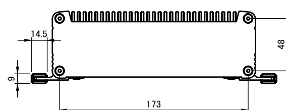
A-A ( 1 : 3.5 )
