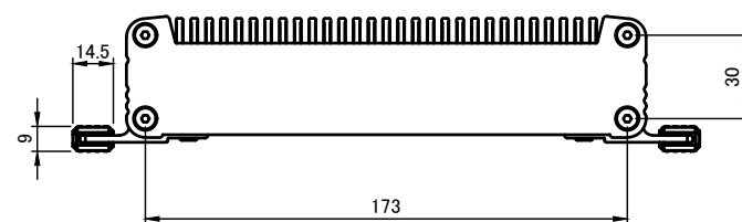
A-A (1:3)
