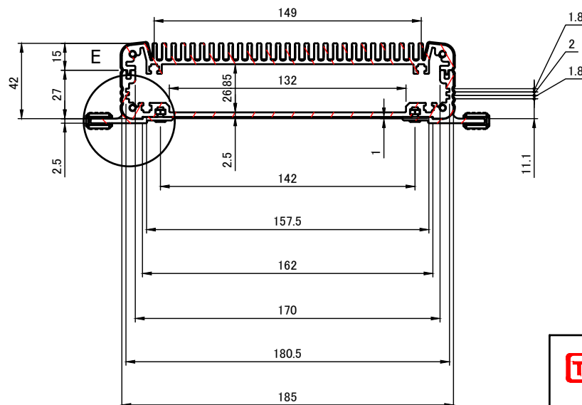
A-A (1:3)
