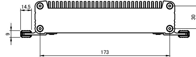
A-A (1:3)
