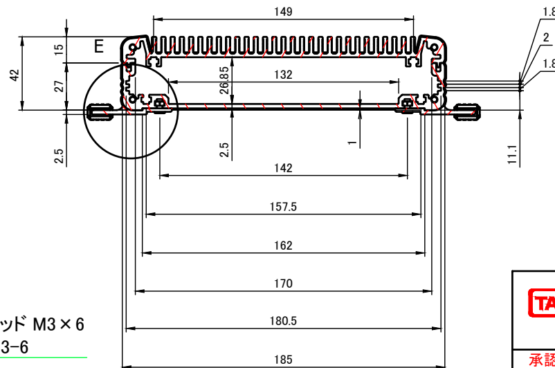
A-A (1:3)
