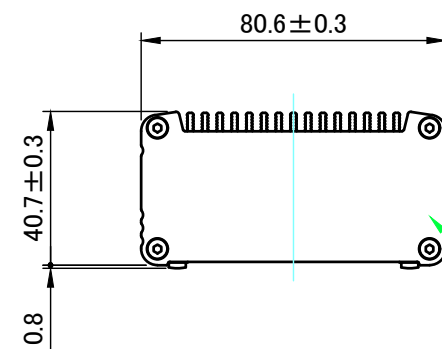
B-B (1:2)
