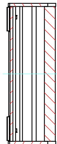
A-A ( 1 : 1.5 )
