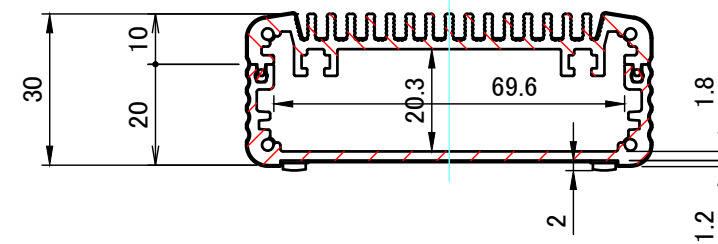
B-B ( 1 : 1.5 )
