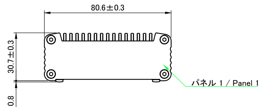
B-B ( 1 : 1.5 )
