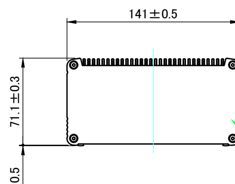
B-B ( 1 : 3 )
