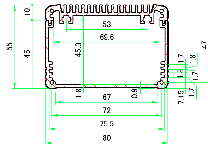
A-A (1:1.5)
