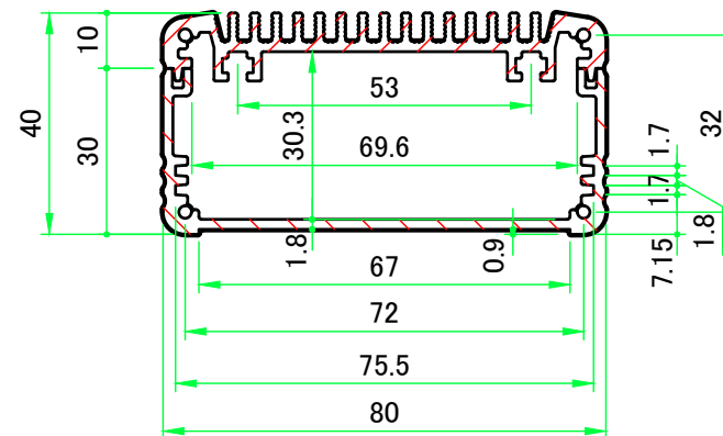
A-A (1 : 1.5)
