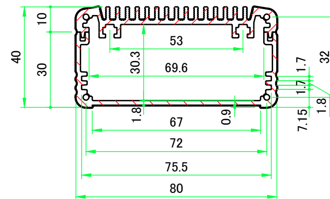
A-A (1:1.5)
