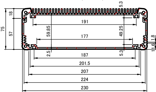
A-A ( 1 : 4 )
