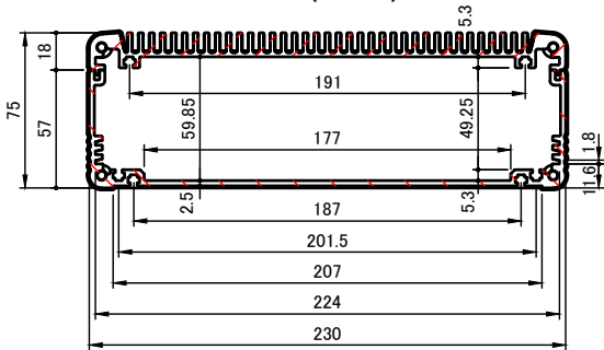
A-A ( 1 : 4 )
