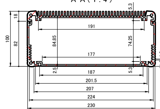
A-A (1:4)
