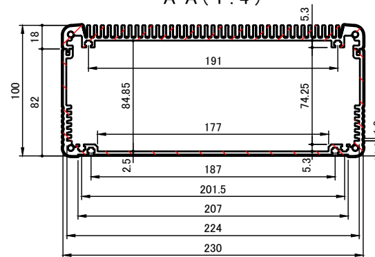
A-A (1:4)
