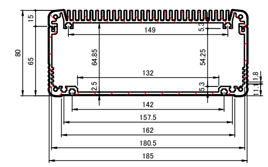
A-A ( 1 : 3.5 )
