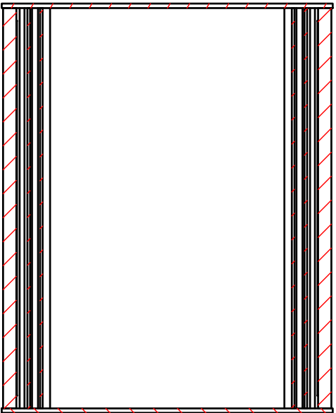
D-D ( 1 : 3 )
