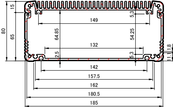
A-A ( 1 : 3 )
