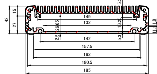
A-A ( 1 : 3.5 )
