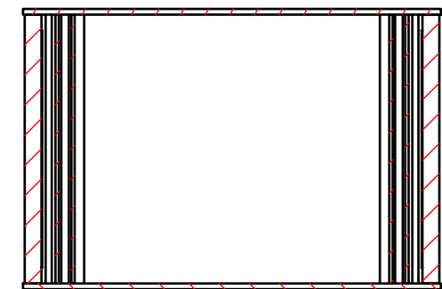
D-D (1:3)
