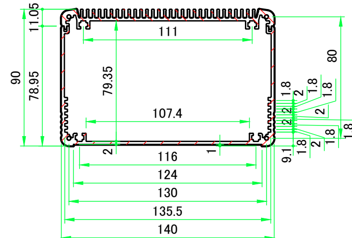
A-A ( 1 : 2.5 )
