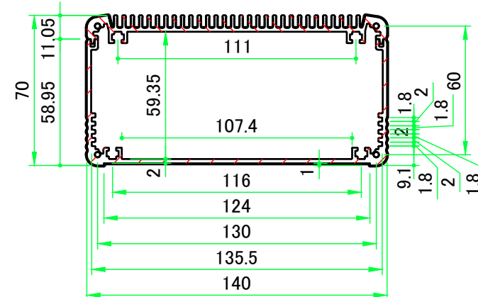
A-A (1:2.5)
