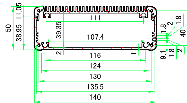
A-A ( 1 : 2.5 )
