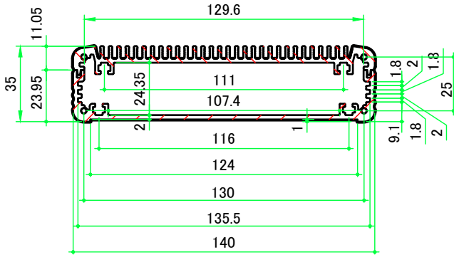
A-A ( 1 : 2.5 )
