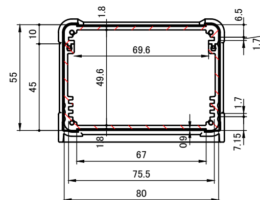
A-A (1:2)
