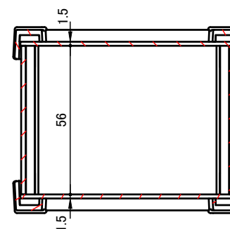
C-C (1:2)
