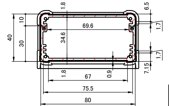
A-A (1:2)
