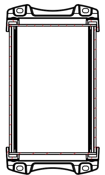
D-D (1:2)
