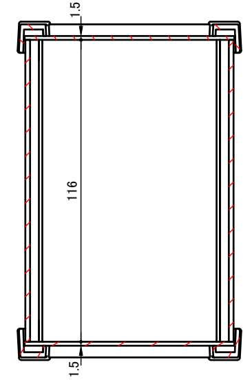
C-C (1:2)
