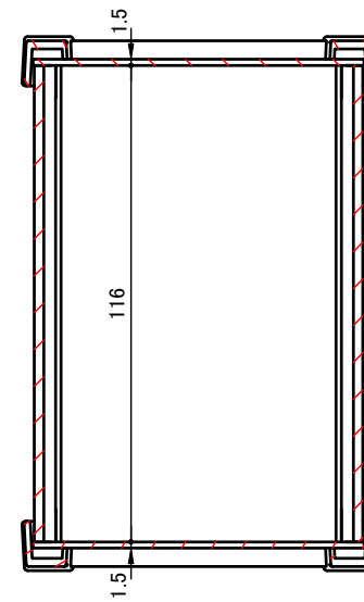
C-C (1:2)
