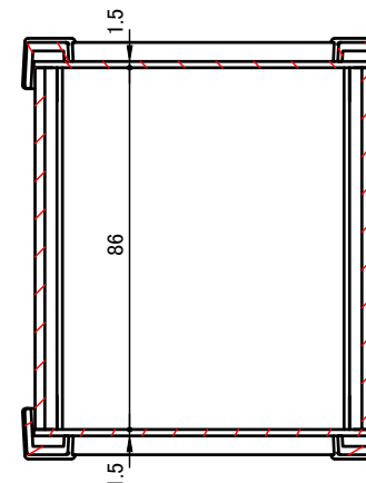
C-C (1:2)
