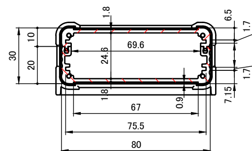
A-A (1:2)
