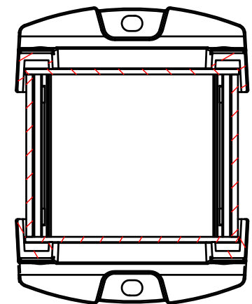
D-D ( 1 : 1.5 )
