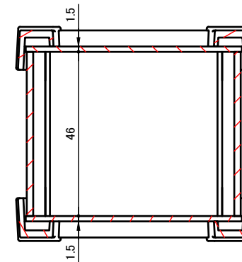
C-C ( 1 : 1.5 )
