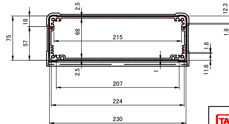
A-A ( 1 : 4 )
