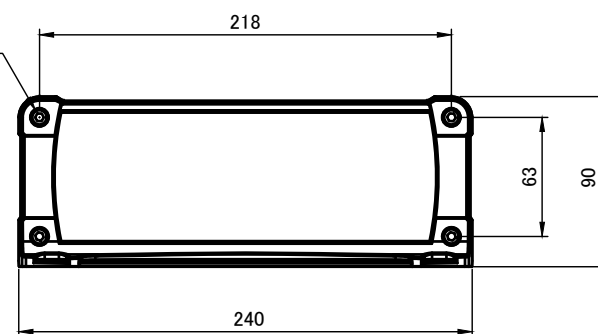
A-A (1:4)
