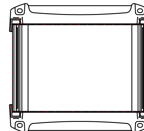
D-D (1:4)
