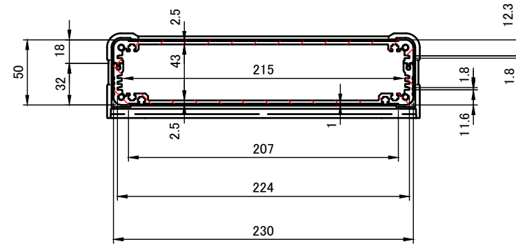
A-A (1:4)
