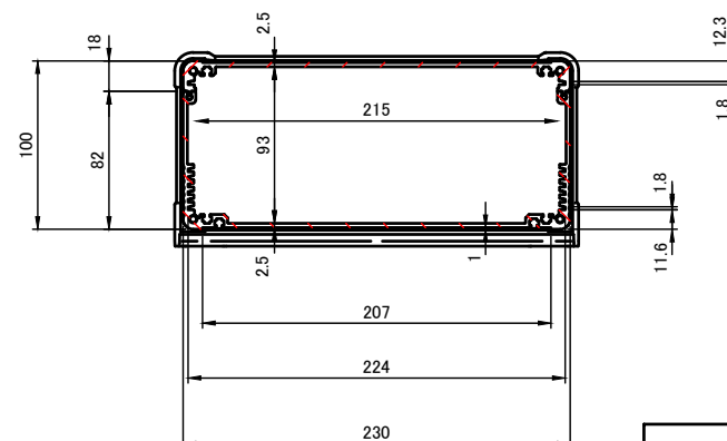
A-A (1:5)
