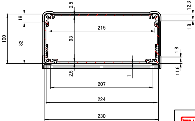
A-A (1:4)
