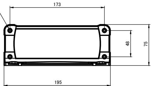
A-A (1:4)
