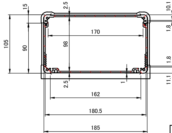
A-A (1:4)
