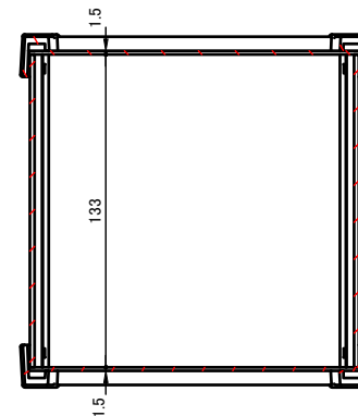
C-C (1:3.5)
