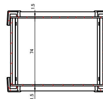
C-C ( 1 : 2.5 )
