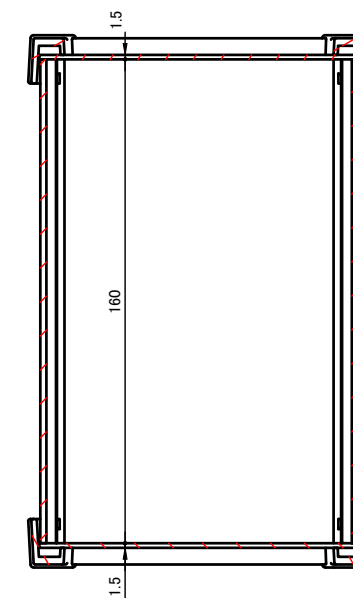
C-C ( 1 : 2.5 )
