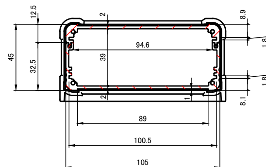
A-A ( 1 : 2.5 )
