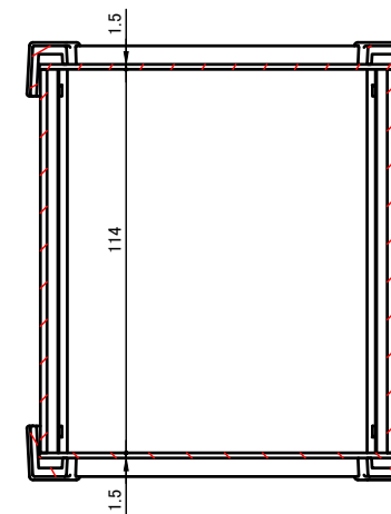
C-C ( 1 : 2.5 )
