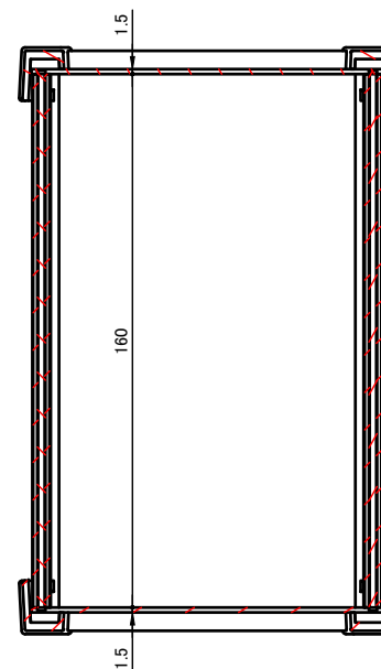
C-C ( 1 : 2.5 )
