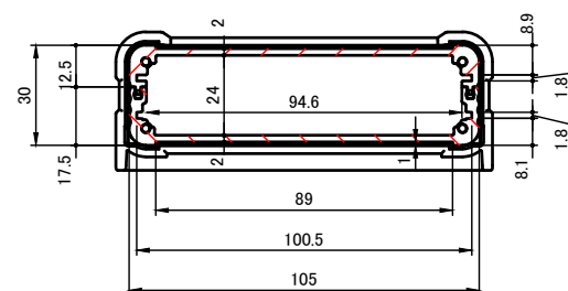
A-A (1:2.5)
