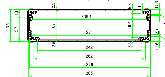
A-A (1:5)
