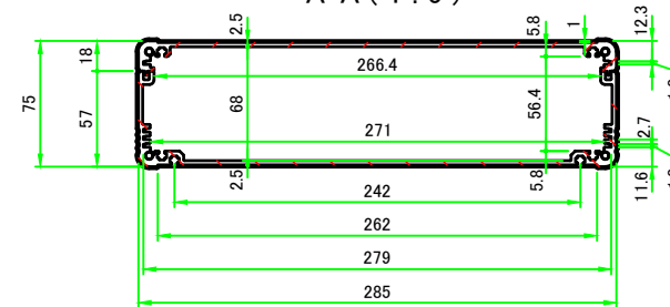
A-A (1:5)
