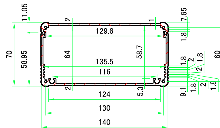
A-A ( 1 : 2.5 )
