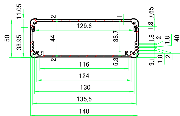
A-A ( 1 : 2.5 )
