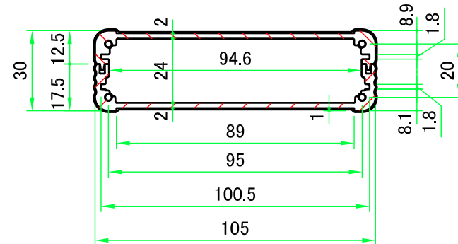
A-A ( 1 : 2 )
