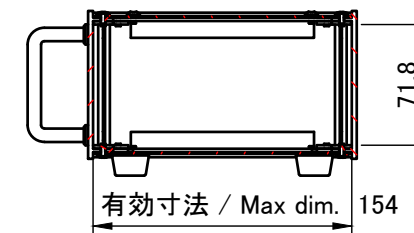
A-A (1:4.5)
