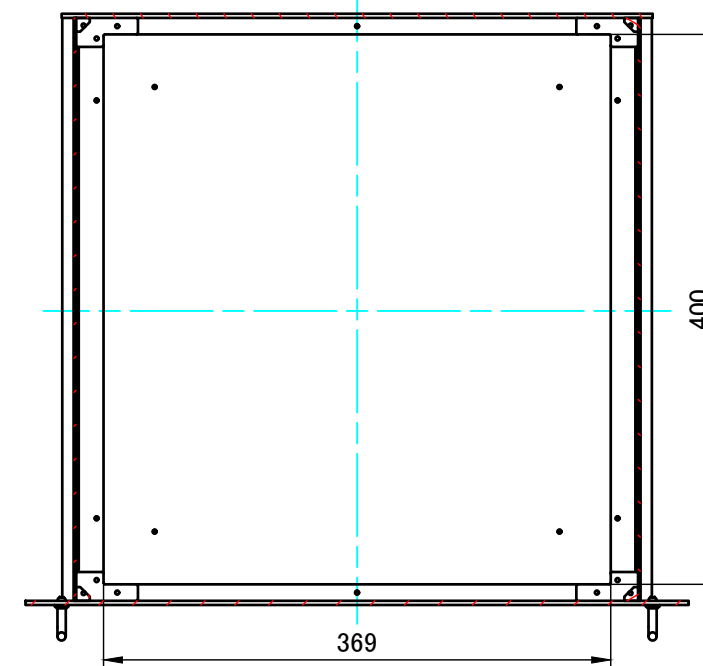
B-B ( 1 : 5.5 )
