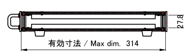
A-A (1:5)
