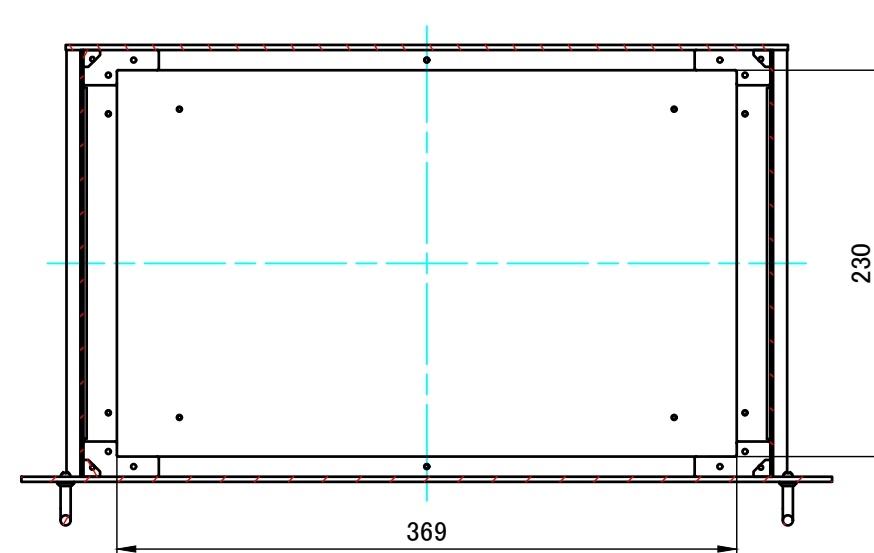
B-B ( 1 : 4.5 )
