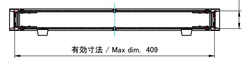
C-C (1 : 4.5)
