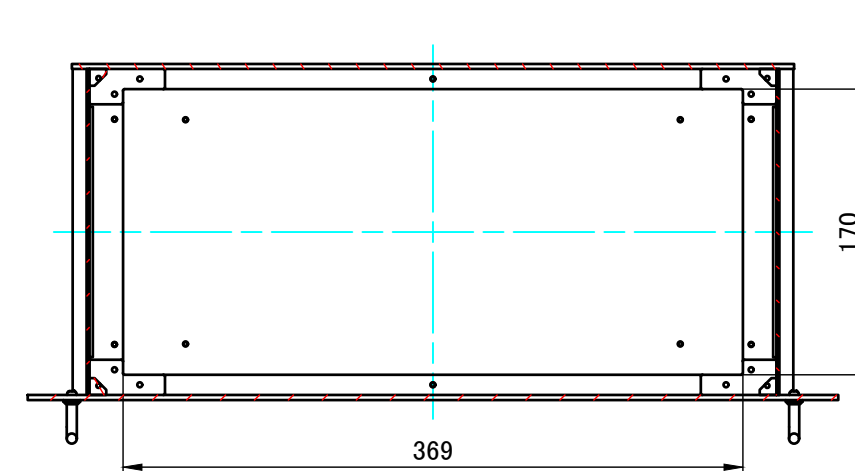
B-B (1 : 4.5)
