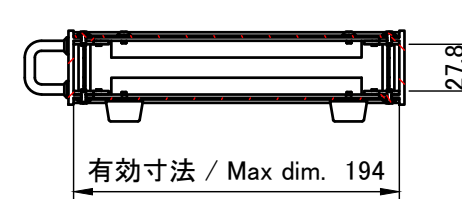
A-A (1 : 4.5)
